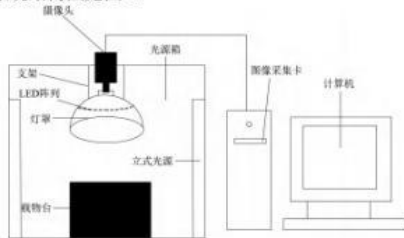
图1 鲷鱼视觉图像采集系统
